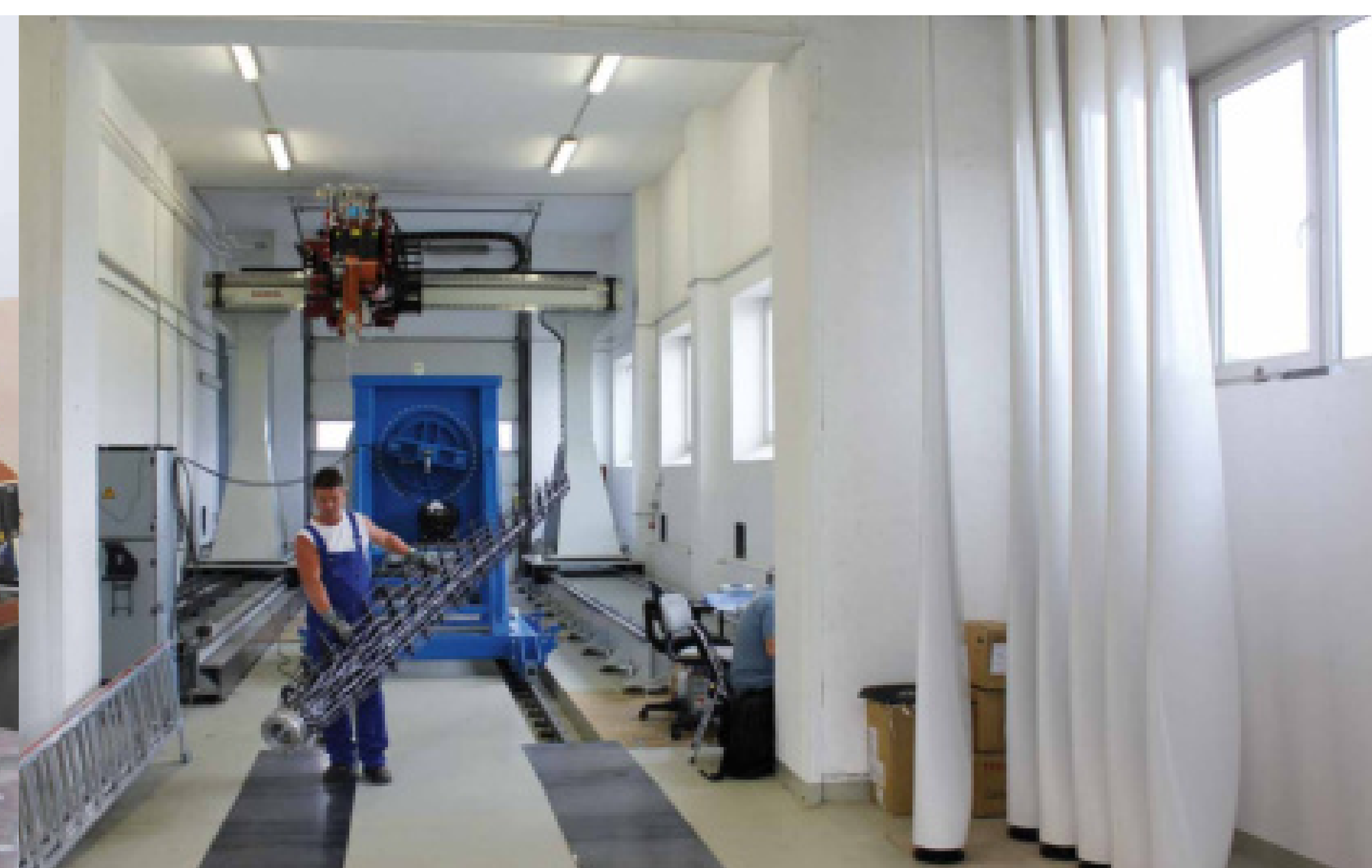
Rotorblattfertigung Rotor blade construction
